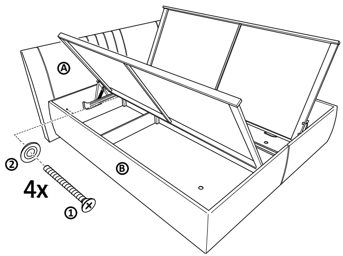
b) Upevnenie čela postele o kontajnery s bočným výklopom roštu
